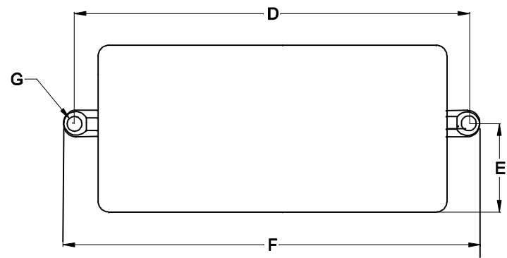
VISTA INFERIOR
